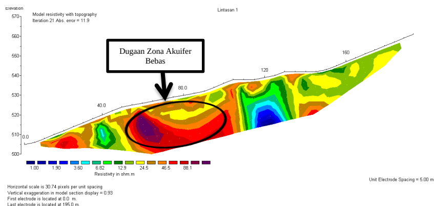
Gambar 3. Penampang 2D Lintasan 1 dengan Topografi
