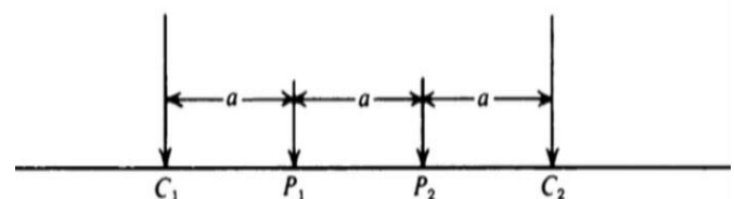
Gambar 1. Susunan elektroda konfigurasi Wenner (Telford et al., 1990).
